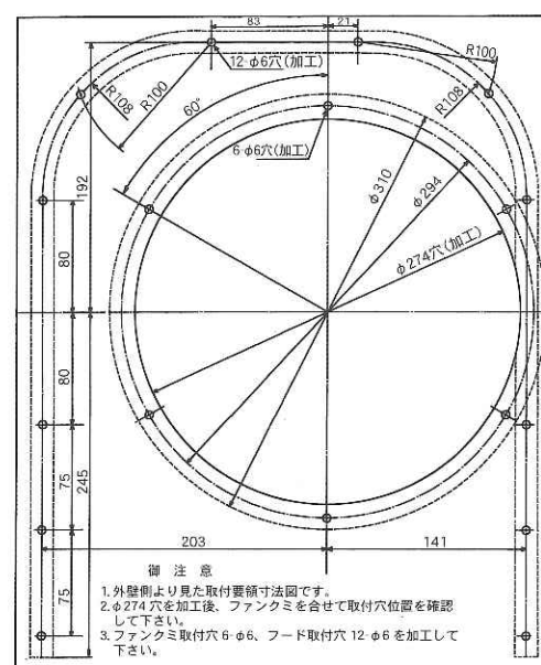
取付要領寸法図
